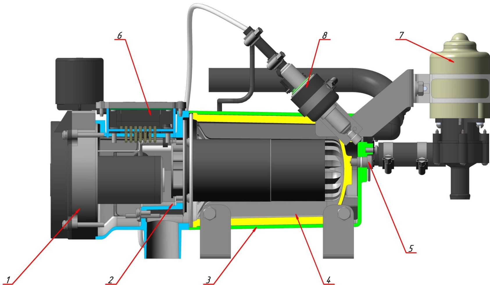
Рисунок 1 Схема деления подогревателя
